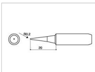
900L-T-I Shape-I
