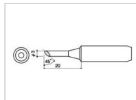
900L-T-3C Shape-3C
