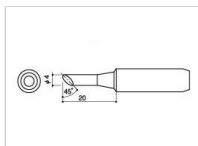
900L-T-4C Shape-4C
